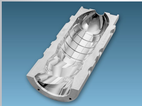
Im Röders-Blasformenbau aus dem Rohblock auf der Maschine mit Emulsion hergestellte und vermessene Blasform
