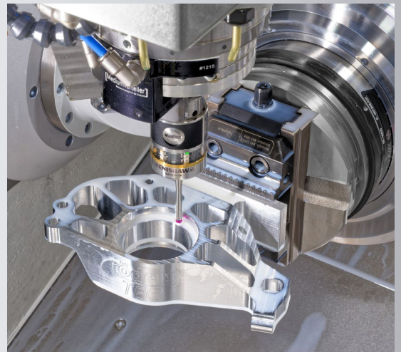
Qualitätskontrolle direkt in der Maschine: Vermessung eines Werkstücks nach der Bearbeitung
