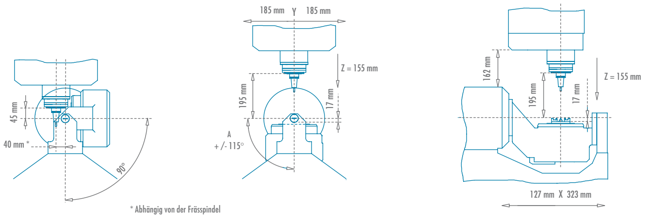
Einspindelmaschine mit schnellem Werkzeugwechsler
